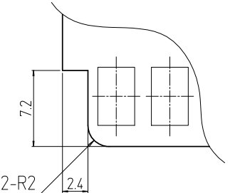
A部詳細 (2 : 1) (反対側も同加工)
