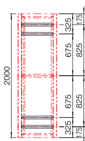
標準取付位置 ラック内部
