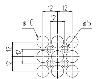
パンチング部詳細 (1 : 2) 開口率 約68%
