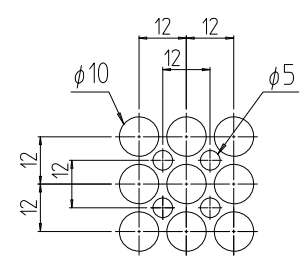
パンチング部詳細 (1 : 2) 開口率 約68%
