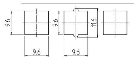
A部詳細 (1 : 1)
