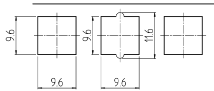
A部詳細 (1:1)
