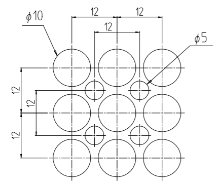
パンチング部詳細 (1 : 1) 開口率 約68%
