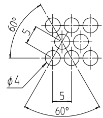
パンチング穴詳細 (1 : 1)
