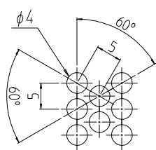
パンチング穴詳細 (1 : 1)
