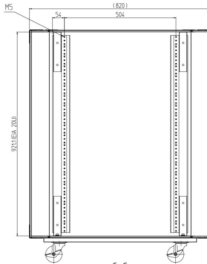
C-C
