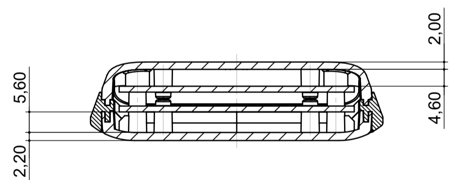
Schnitt B-B
