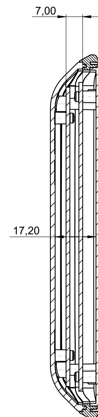
Schnitt A-A
