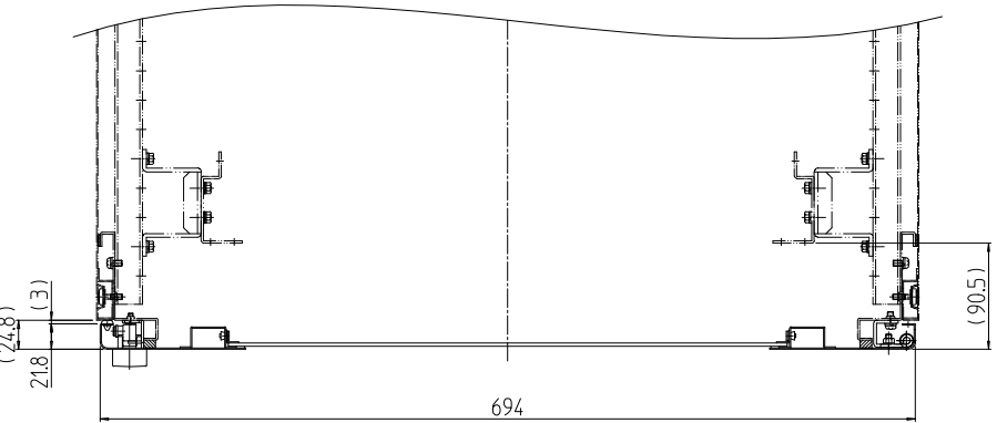
A-A (1 : 7)
