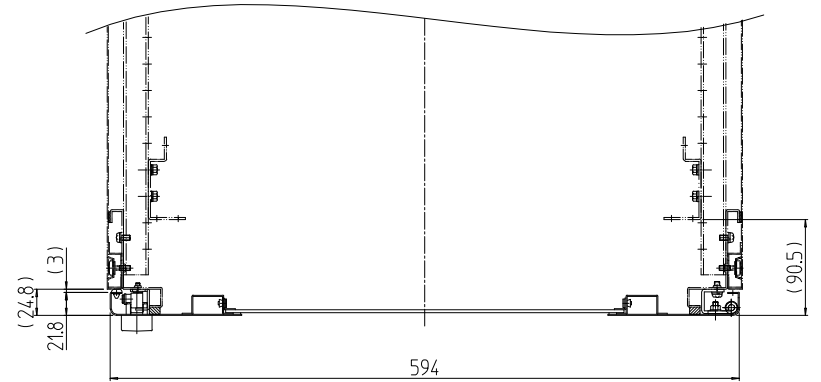
A-A (1 : 7)
