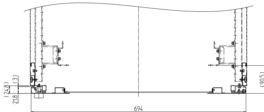
A-A (1 : 7)
