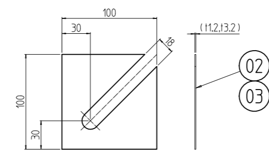
架台用ライナー外観寸法 (1 : 4)
