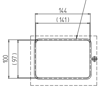
A部詳細 (1 : 6)
