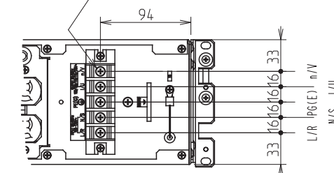
INSIDE VIEW OF TB COVER (REAR) TBカバー内部 (背面)
