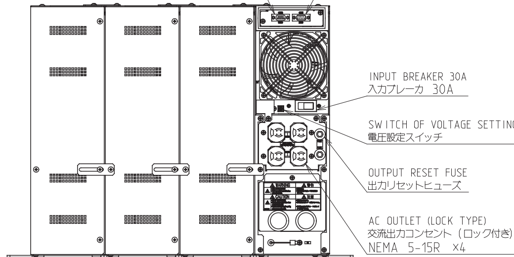
REAR VIEW 背面
