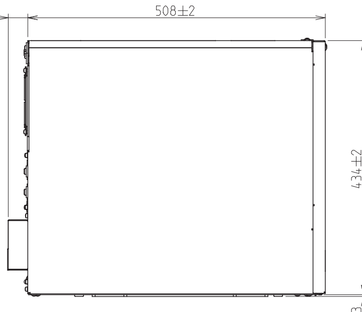
LEFT SIDE VIEW 左側面
