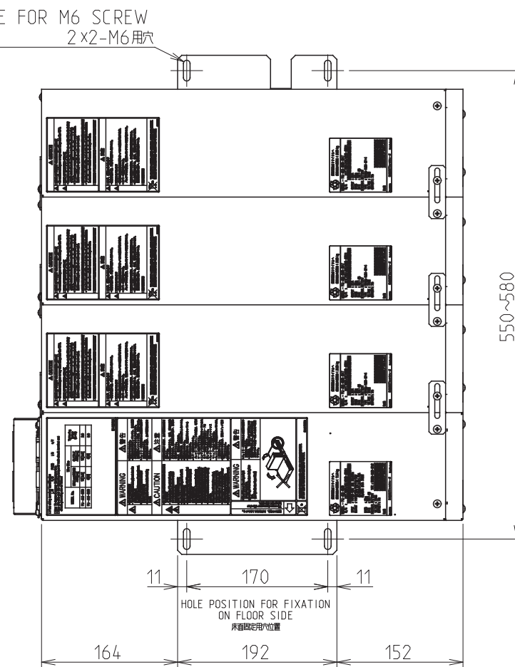
TOP VIEW 平面
