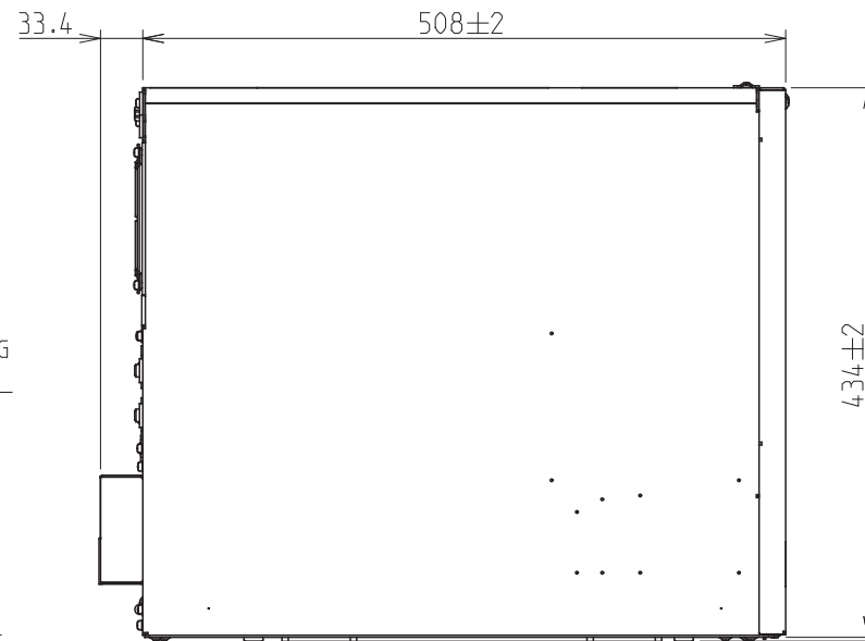
LEFT SIDE VIEW 左側面
