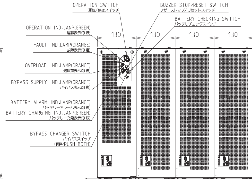
FRONT VIEW 正面
