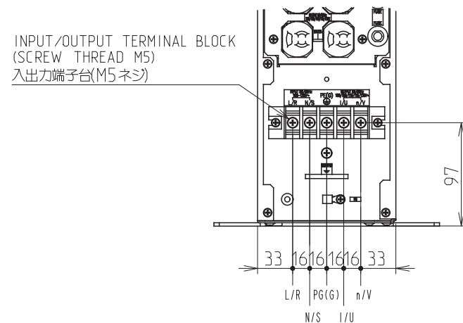
INSIDE VIEW OF TB COVER TBカバー内部
