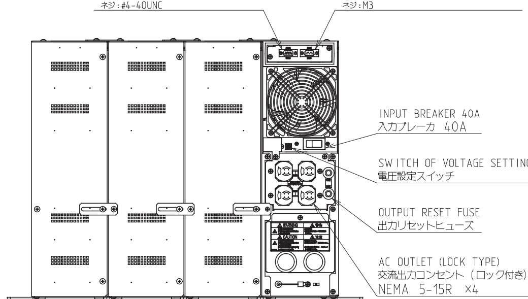
REAR VIEW 背面
