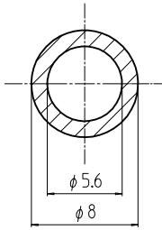
A-A (2:1)
