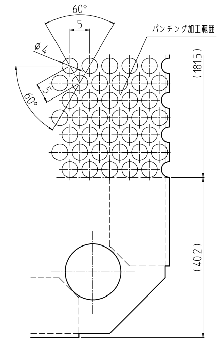
A部詳細 (1 : 1)
