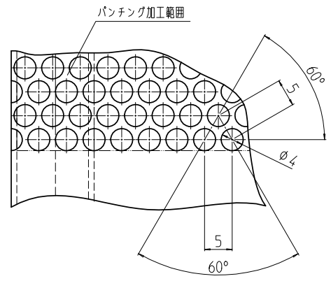
A部詳細 (1 : 1)
