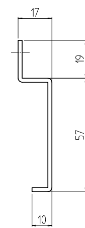
A-A (1 : 2)
