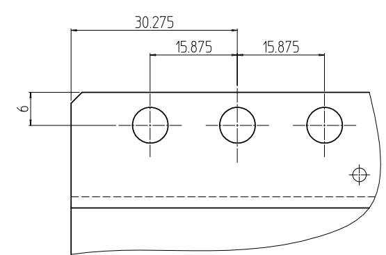
B部詳細 (1 : 1) (42カ所同様に加工)
