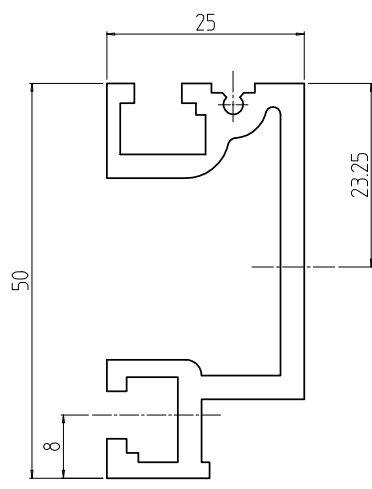
A-A (1 : 1)
