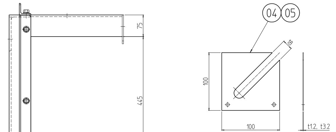
架台用ライナー詳細 (1 : 4)
