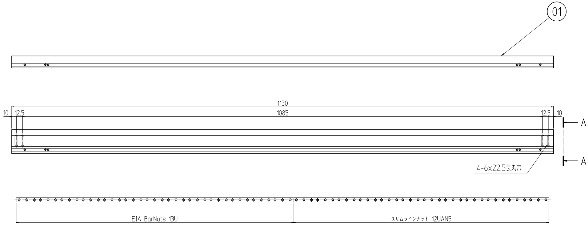
バーナット実装図
