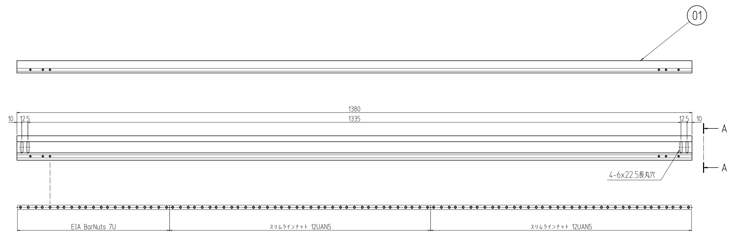
バーナット実装図
