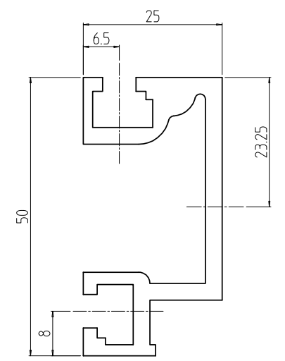
A-A (1 : 1)
