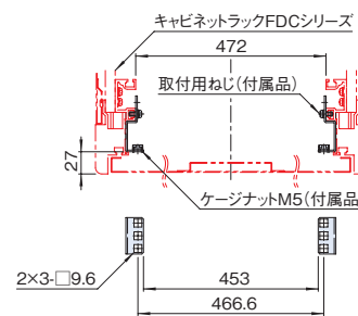
取付例
