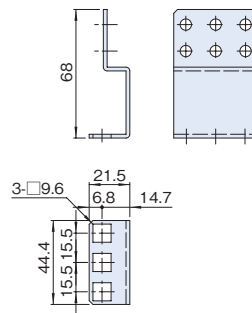
取付例
