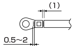
圧着端子カシメ位置寸法
