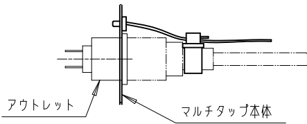
垂直断面図
