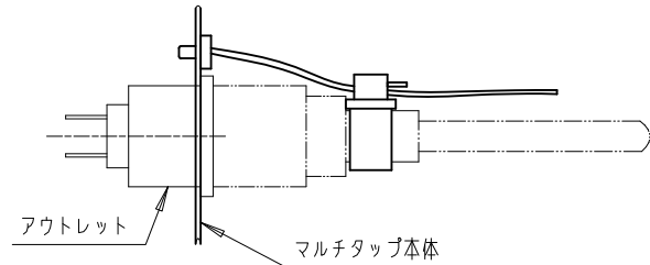
垂直断面図
