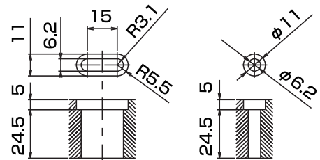
本体取付穴寸法
